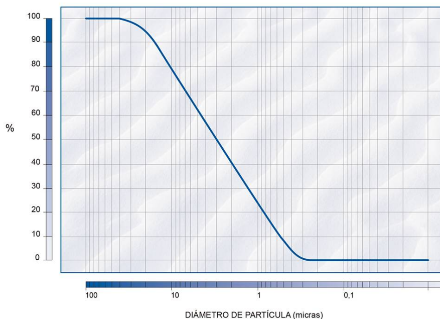
DISTRIBUCIÓN GRANULOMÉTRICA
